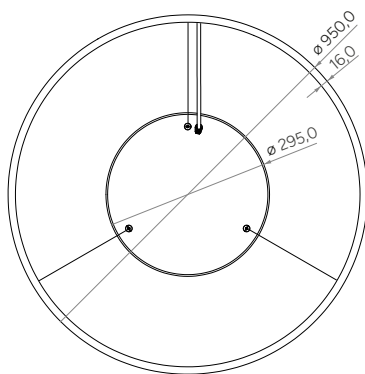
Ring A 950 mm | Widok z góry Ring A 950 mm | Top view
