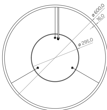
Ring A 600 mm | Widok z góry Ring A 600 mm | Top view
